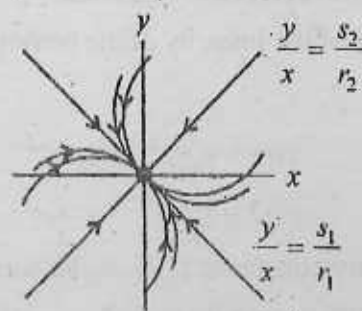
Fig. 6.1 : Stable node
