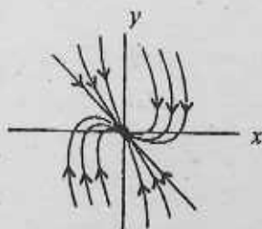
Fig. 6.9 : Phase paths
