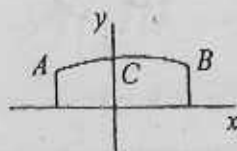
Fig. 6.7 : Phase path
